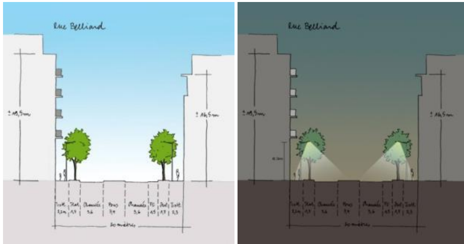
Plantation et adaptation de l'éclairage dans la Rue Belliard (ERU asbl).
