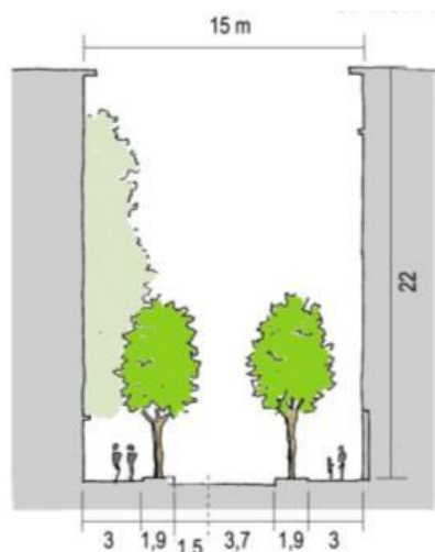
Plantation bilatérale de la Rue de l'Industrie et Rue de la Science (ERU asbl).
